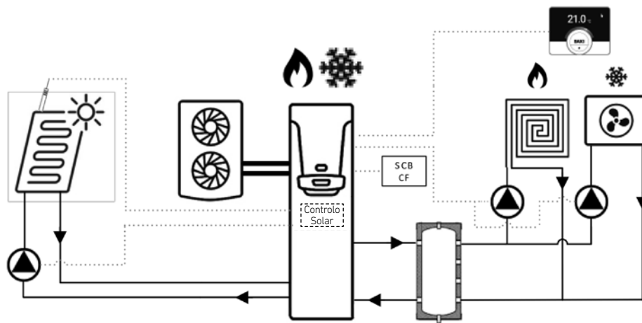
Controlo duma zona, calor por pavimento radiante e frio por ventiloconvetores e controlo de energia solar térmica para pré-aquecimento AQS. Platinum BC iPlus V200 Smart
