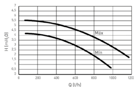
Circulador Gama Platinum Compact ECO Pressão disponível à saída da caldeira
