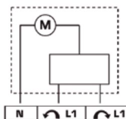
Esquema elétrico
