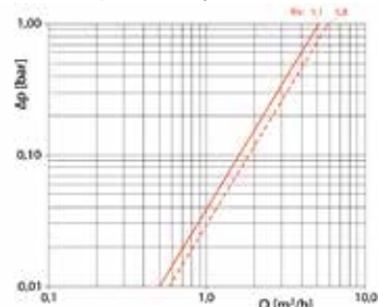
Curva perda de carga
