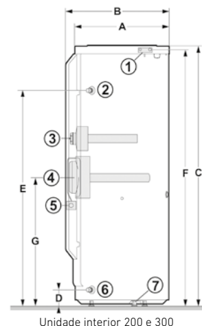
Unidade interior 200 e 300
