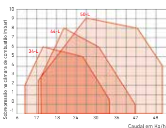
Curvas de caudal pressão
