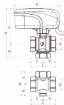
Válvula de zona motorizada com união com fecho
