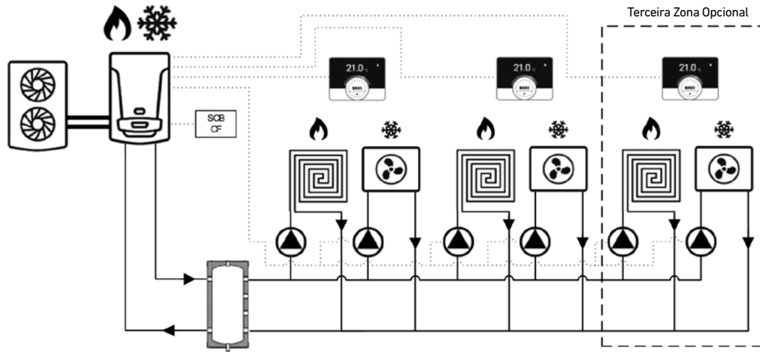
Controlo de três zonas, calor por pavimento radiante e frio por ventiloconvetores, com um circulador por circuito Platinum BC iMax
