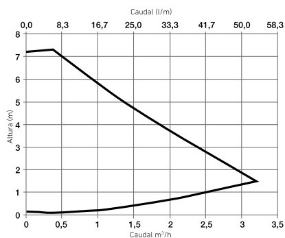
Curva do circulator incluído nos modelos GT, GTF, GTA e GTAF
