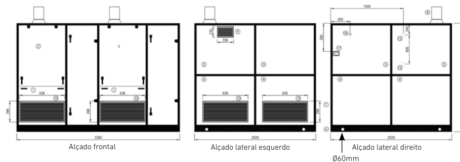
Tipo GME4
