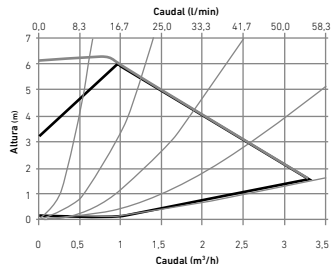
Circulador kit 2º circuito (Ref. 7502759). Pressão disponível à saída da bomba de calor
