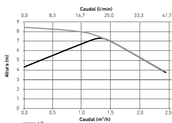
Circulador Platinum BC iMax Pressão disponível à saída da bomba de calor
