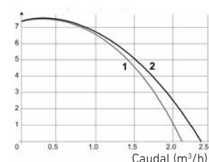
Circulador Argenta Hybrid Pressão (m c.a.)
