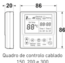
Unidade interior 150
