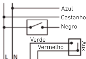
Ligações elétricas
