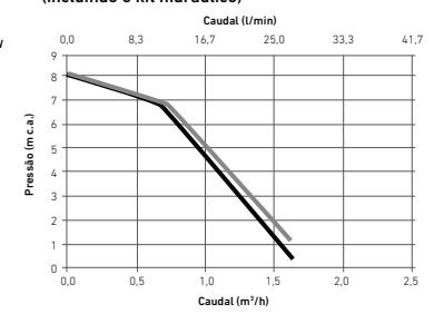
Pressão disponível à saída da bomba de calor (incluindo o kit hidráulico)
