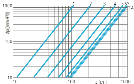
Perda de carga da união com fecho (segundo número de voltas)
