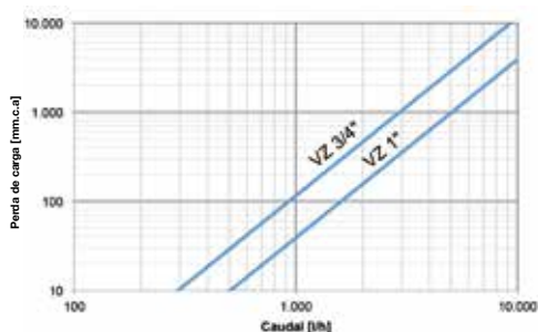
Perda de carga via direta
